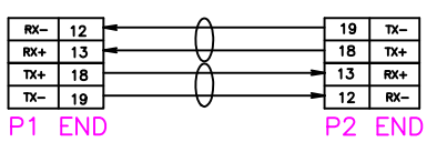
WIRING TABLE
