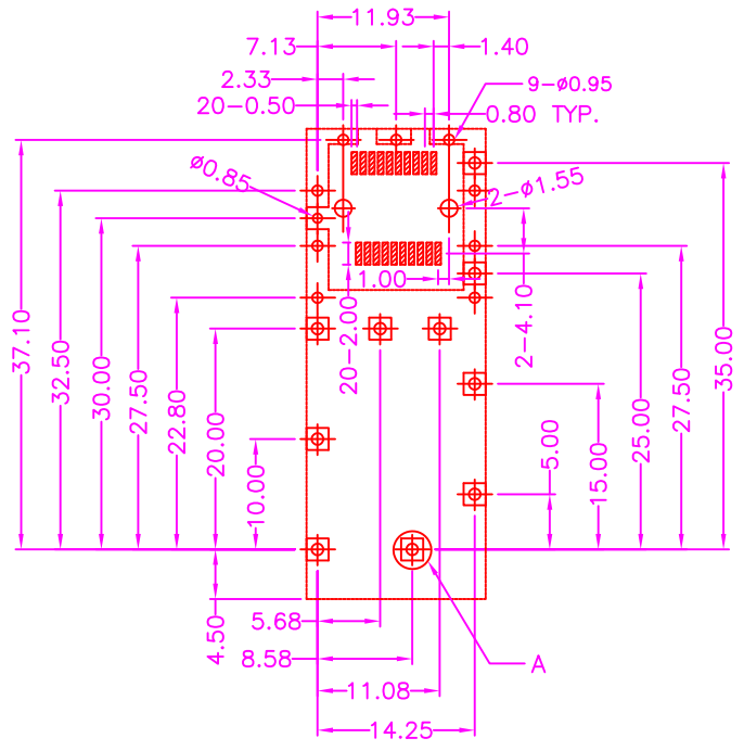
P.C.B LAYOUT TOP VIEW \pm 0.05
