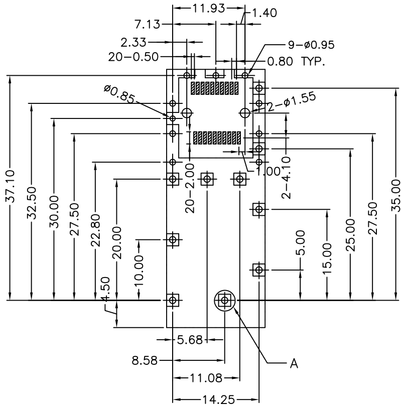
P.C.B LAYOUT TOP VIEW \pm 0.05
