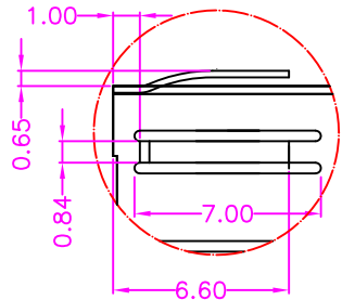
DETAIL: A SCALE: 2.5:1
